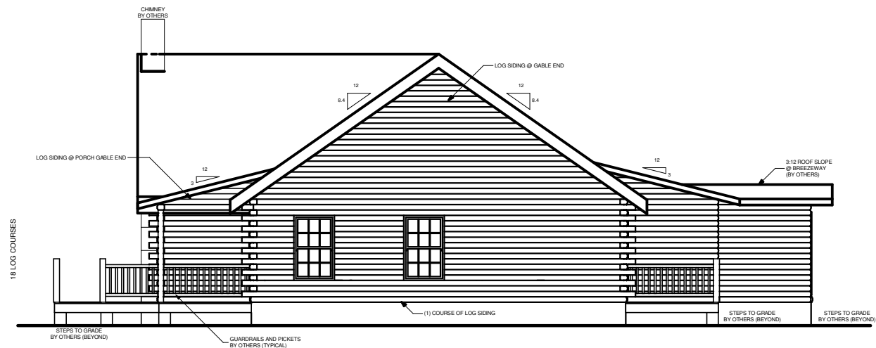
RIGHT ELEVATION
