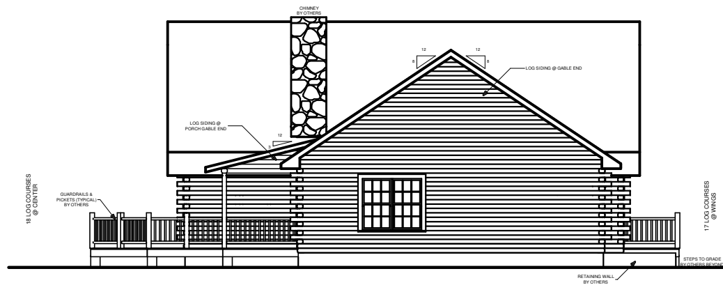
RIGHT ELEVATION
