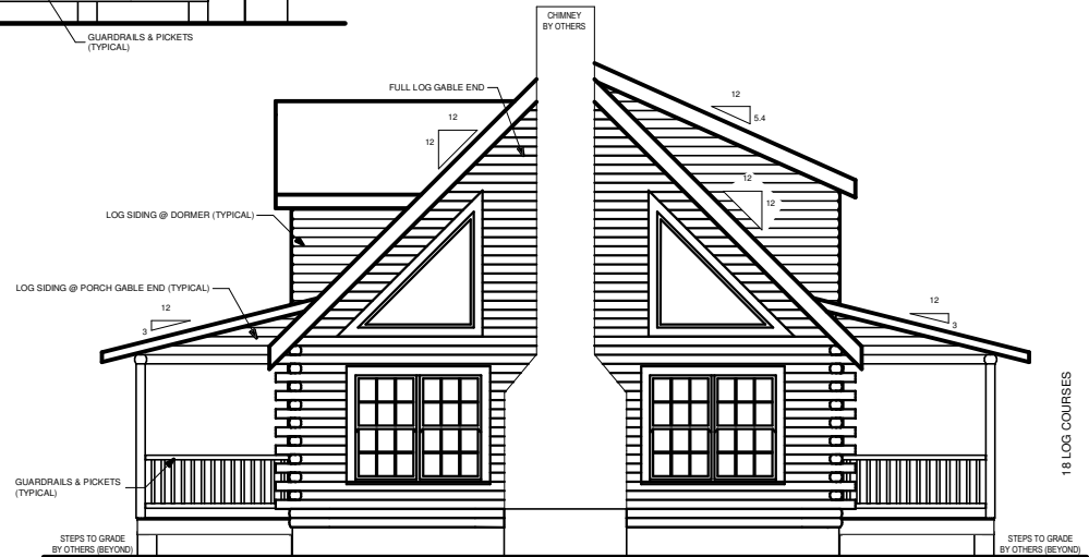
RIGHT ELEVATION
