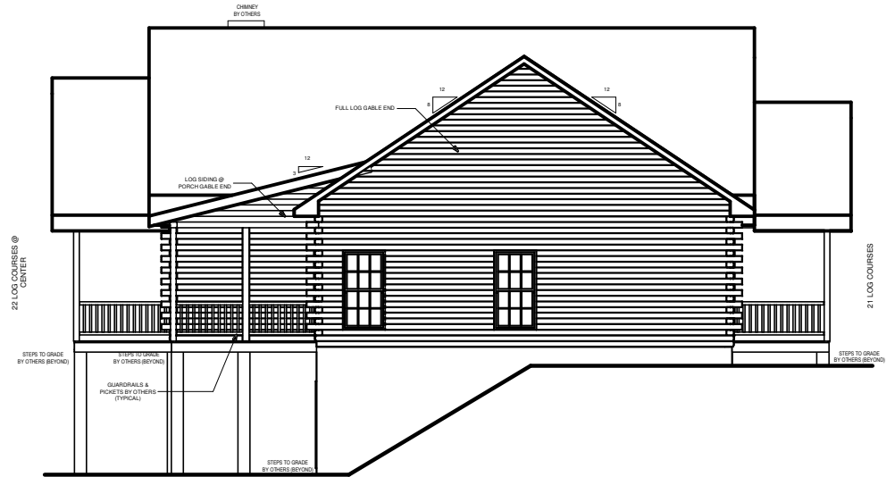
RIGHT ELEVATION
