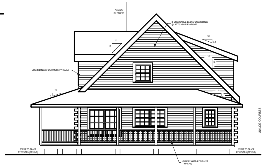
RIGHT ELEVATION
