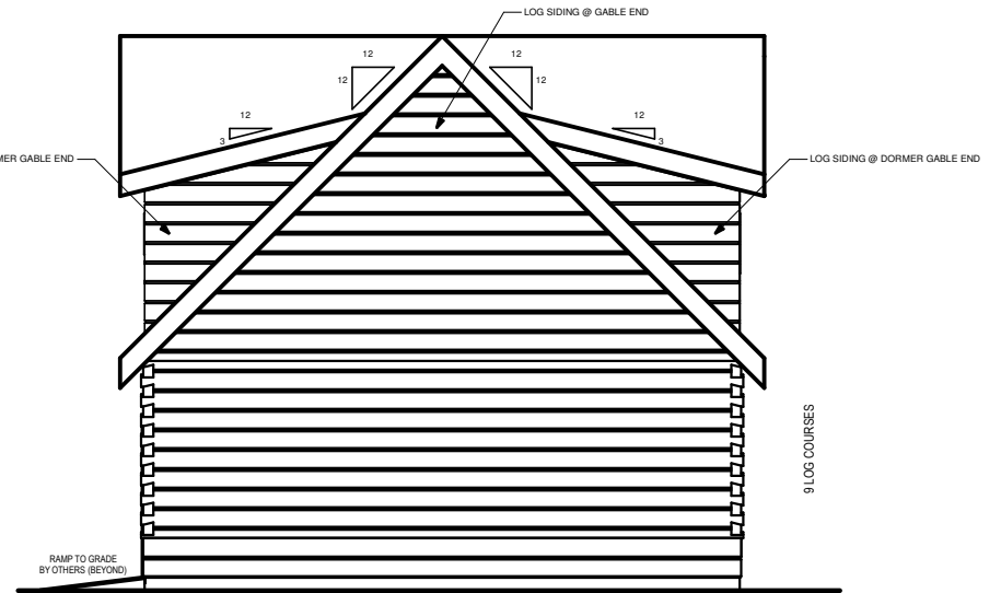
RIGHT ELEVATION
