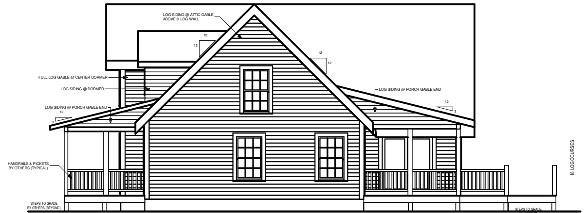
RIGHT ELEVATION
