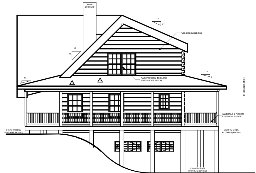
RIGHT ELEVATION
