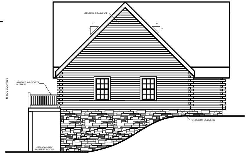
RIGHT ELEVATION
