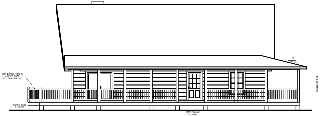
RIGHT ELEVATION
