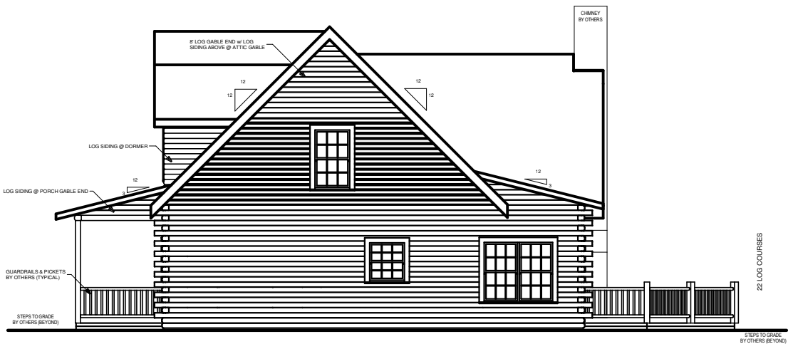
RIGHT ELEVATION
