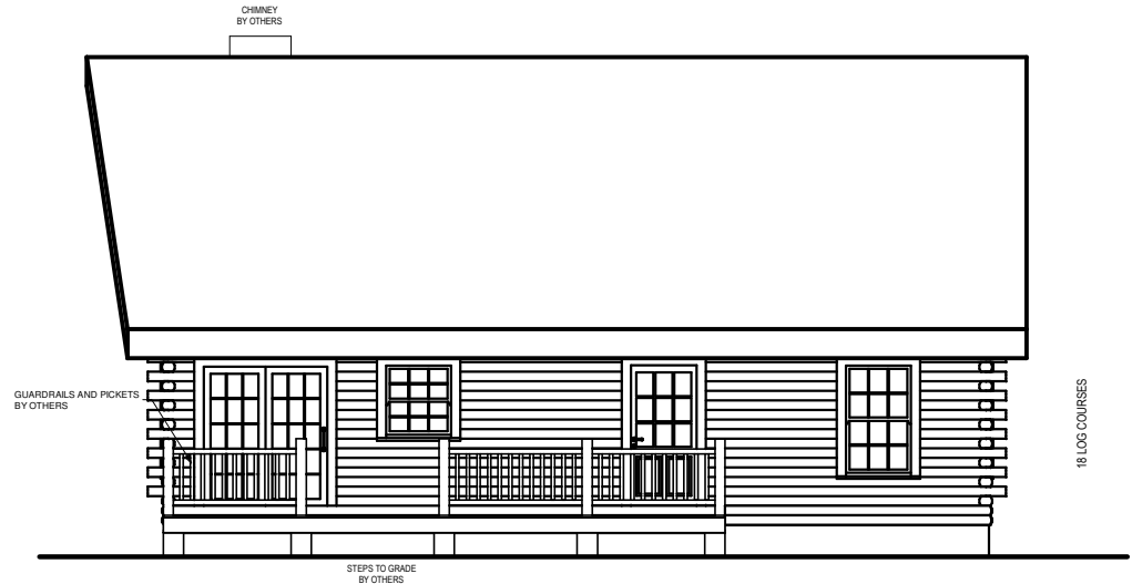
RIGHT ELEVATION
