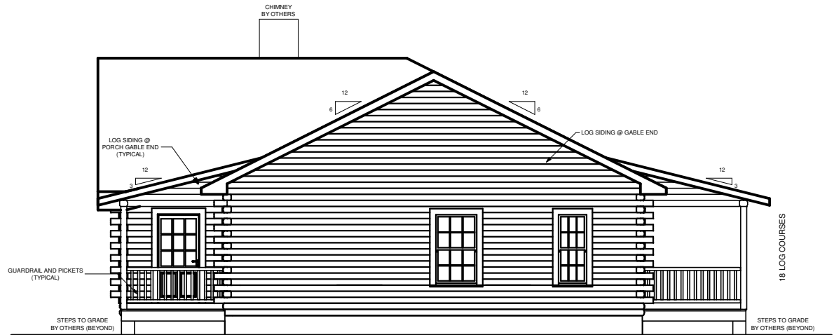
RIGHT ELEVATION
