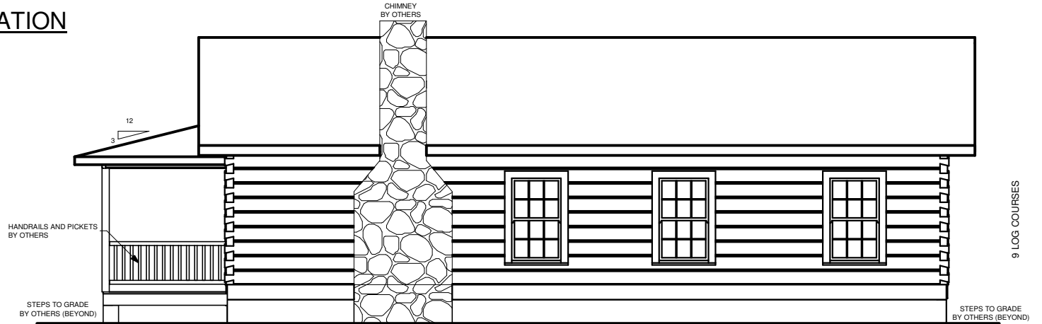
RIGHT ELEVATION
