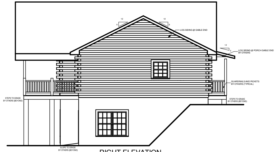
RIGHT ELEVATION
