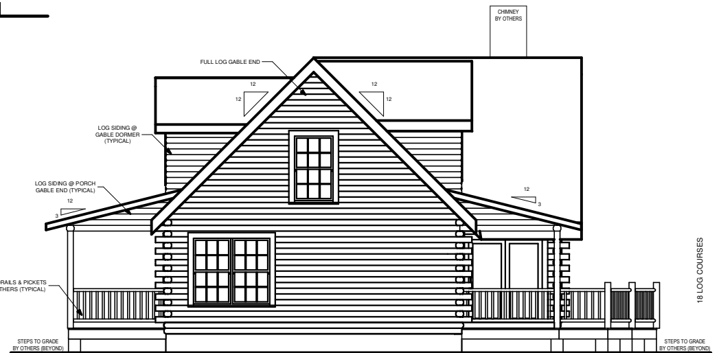
RIGHT ELEVATION
