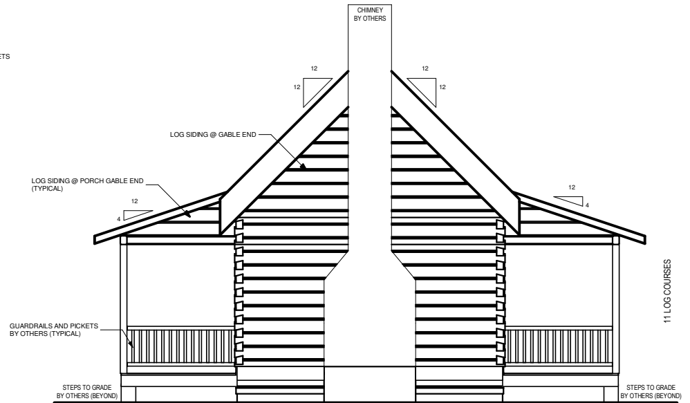
RIGHT ELEVATION
