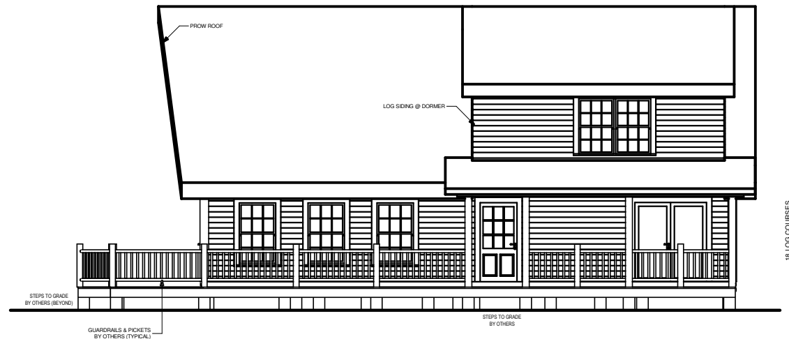
RIGHT ELEVATION
