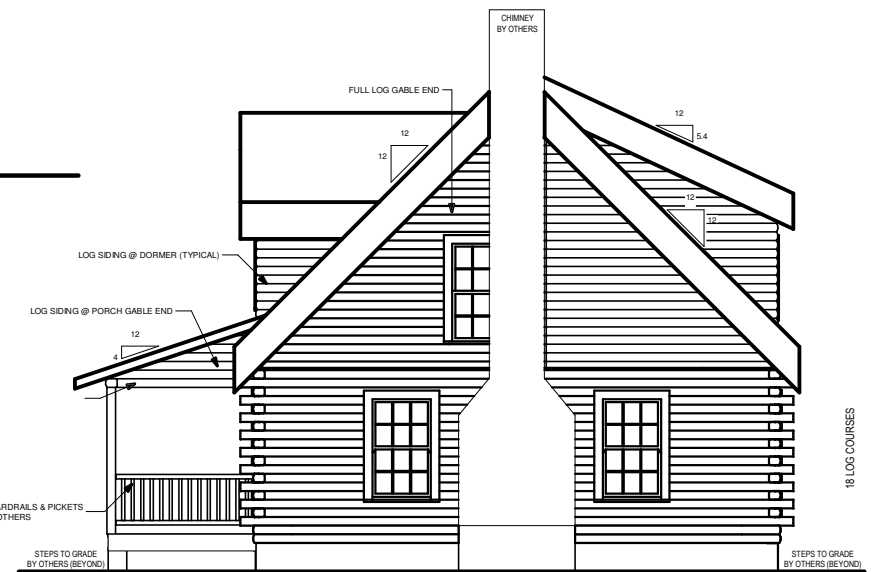
RIGHT ELEVATION
