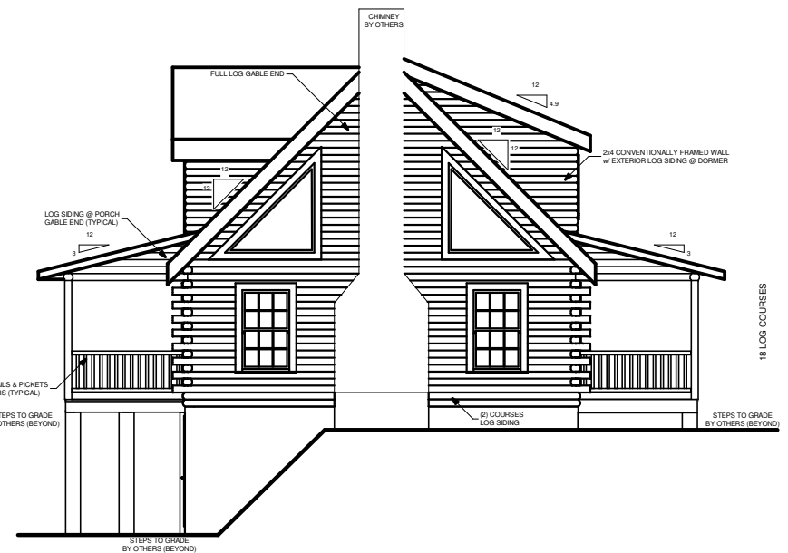
RIGHT ELEVATION
