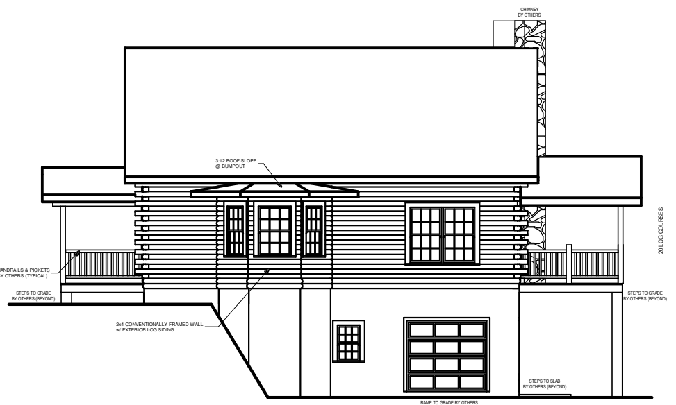
RIGHT ELEVATION
