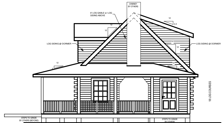
RIGHT ELEVATION
