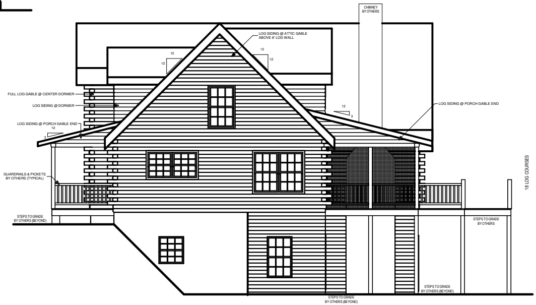
RIGHT ELEVATION
