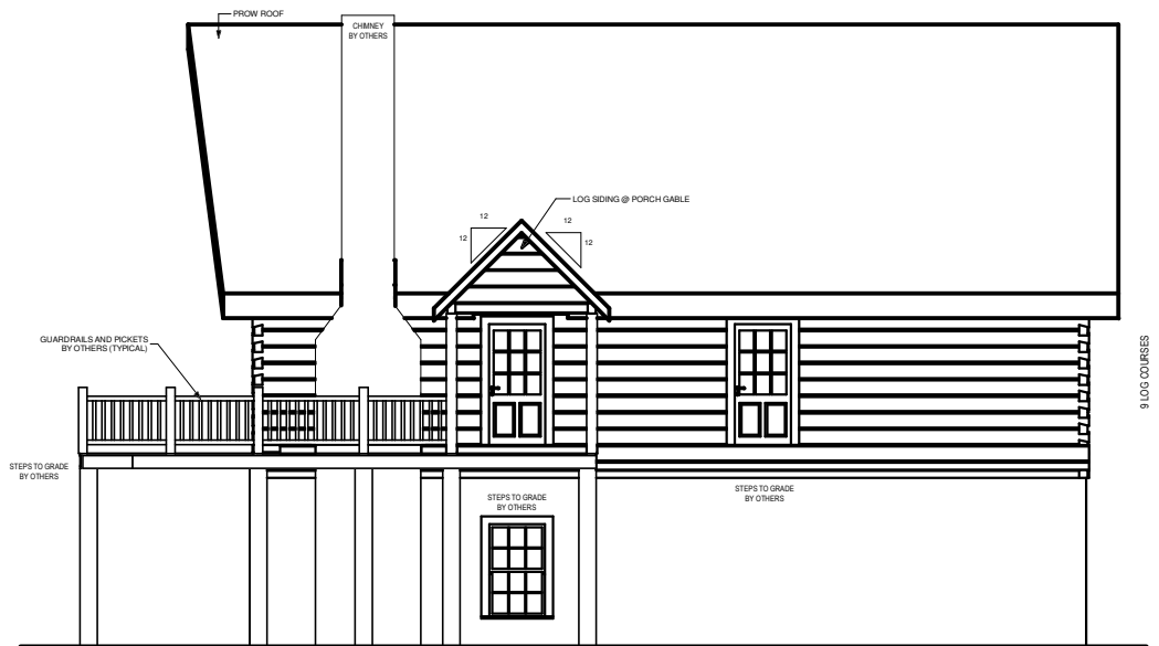
RIGHT ELEVATION
