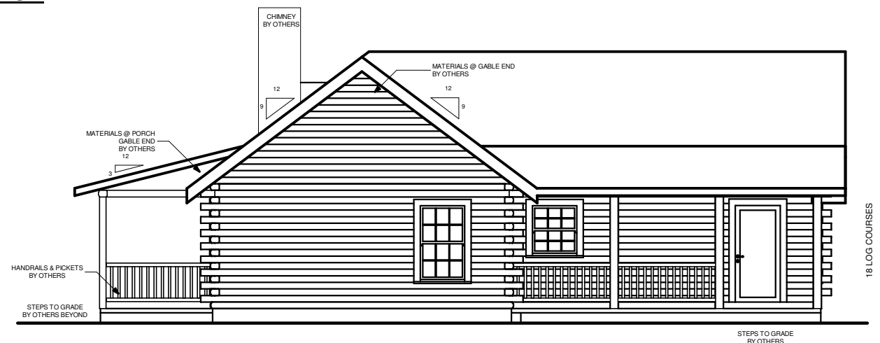
RIGHT ELEVATION
