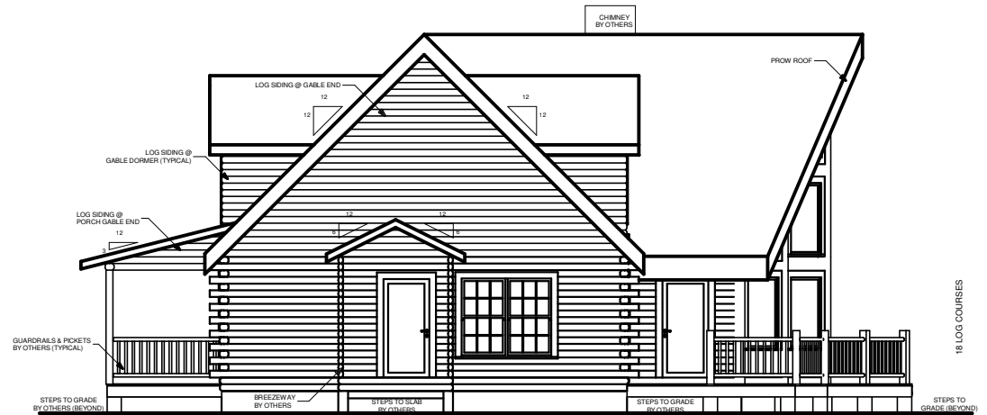
RIGHT ELEVATION
