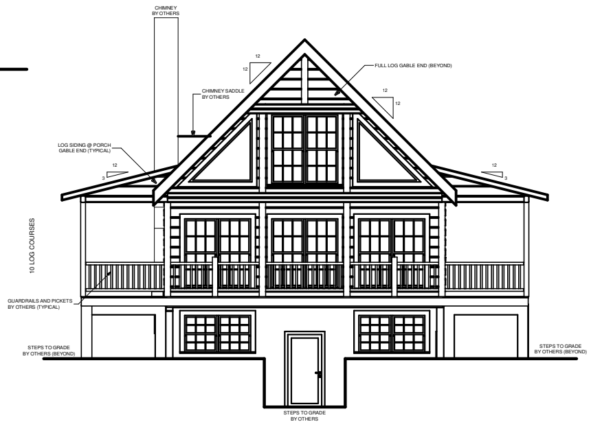
RIGHT ELEVATION
