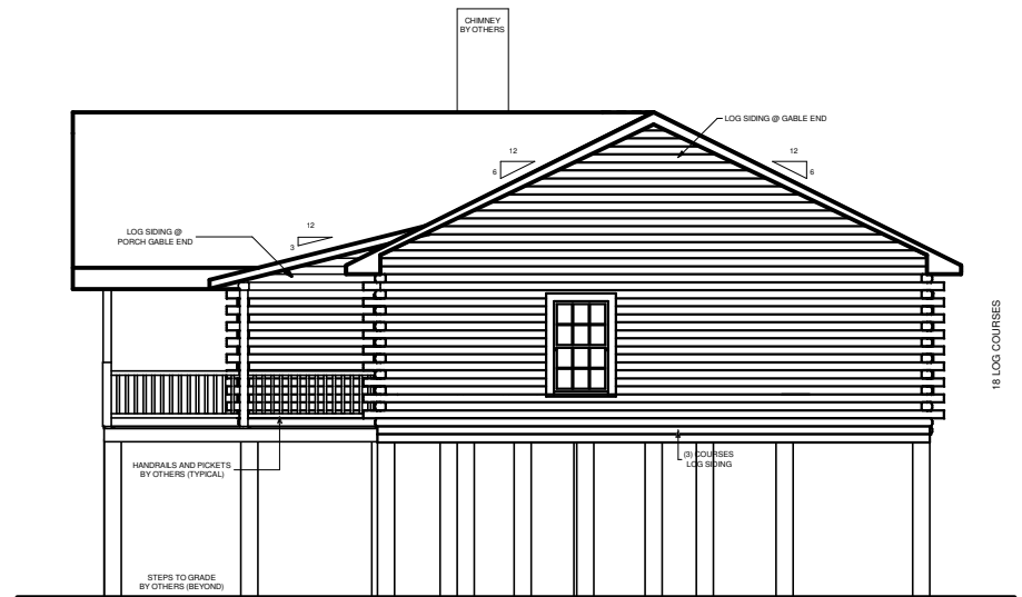
RIGHT ELEVATION
