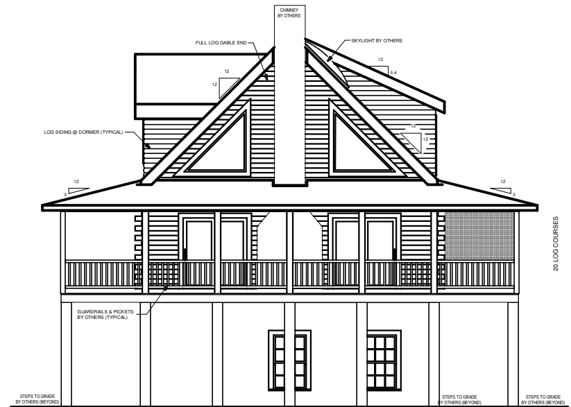
RIGHT ELEVATION
