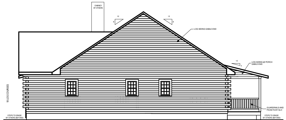
RIGHT ELEVATION
