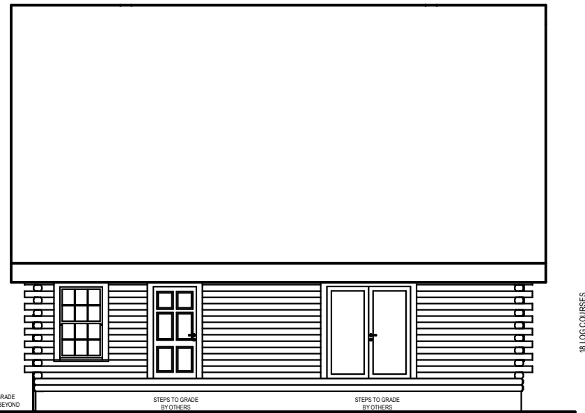
RIGHT ELEVATION
