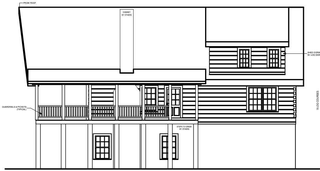
RIGHT ELEVATION
