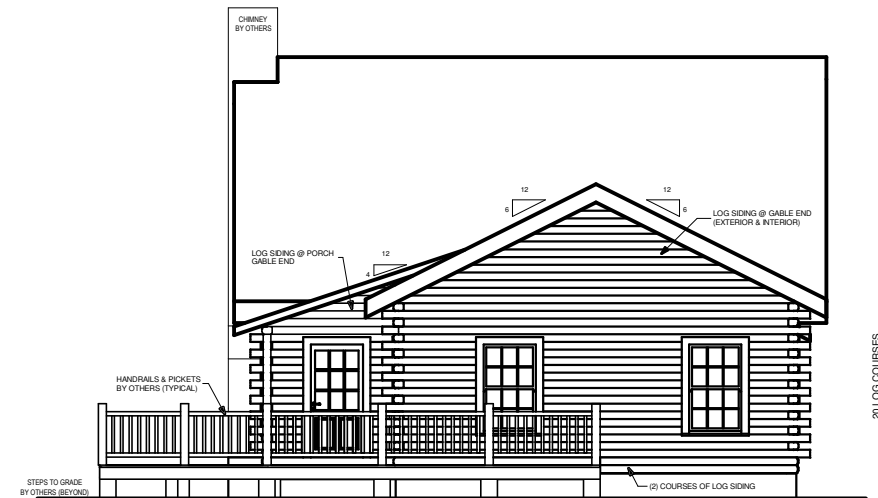
RIGHT ELEVATION
