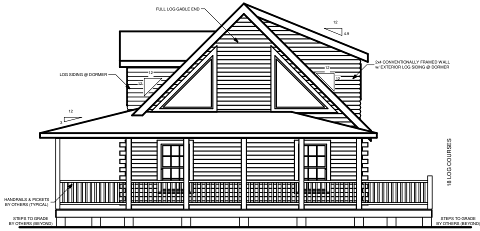
RIGHT ELEVATION
