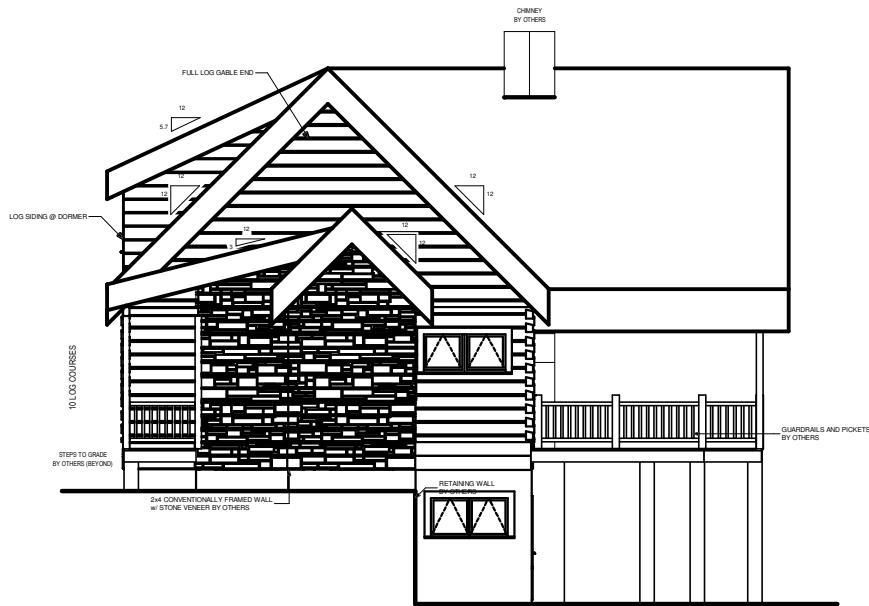
RIGHT ELEVATION
