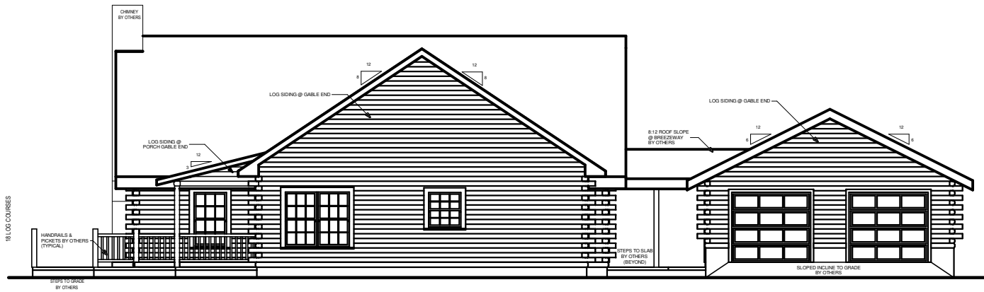
RIGHT ELEVATION
