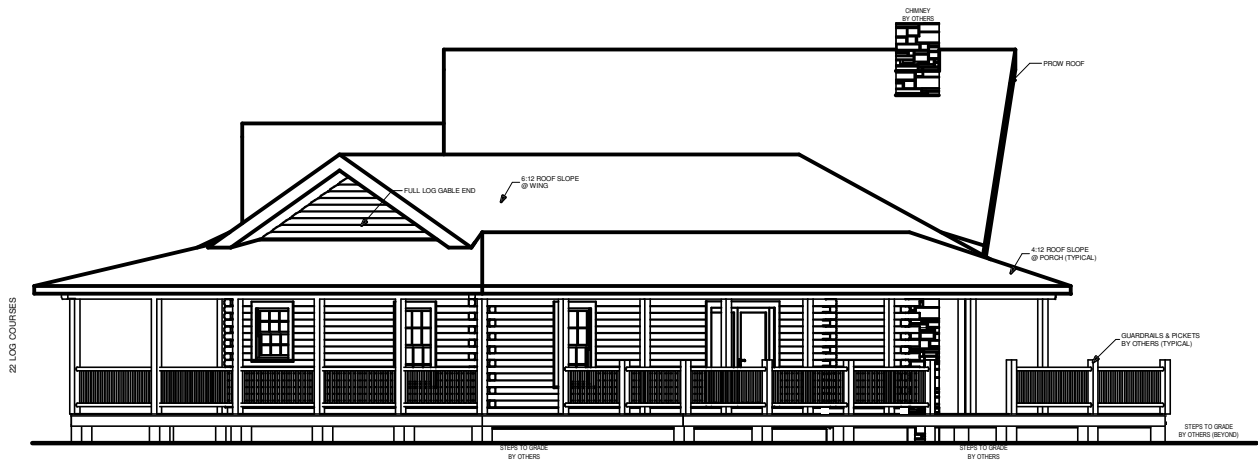
RIGHT ELEVATION
