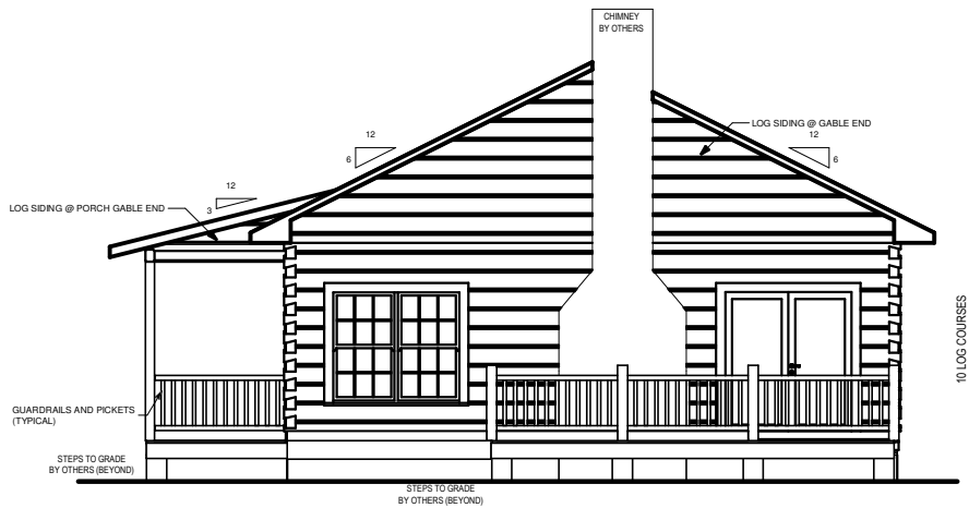
RIGHT ELEVATION
