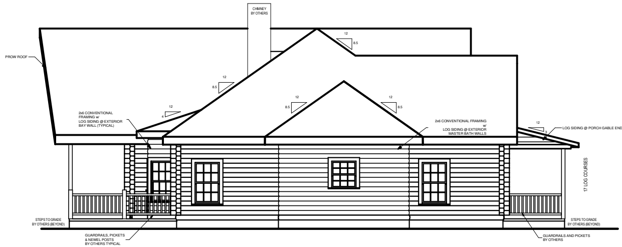
RIGHT ELEVATION
