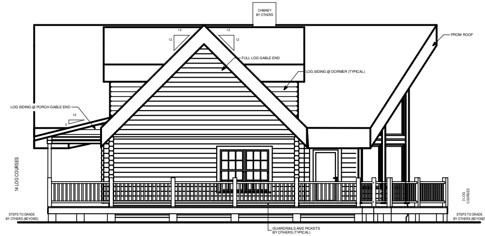
RIGHT ELEVATION
