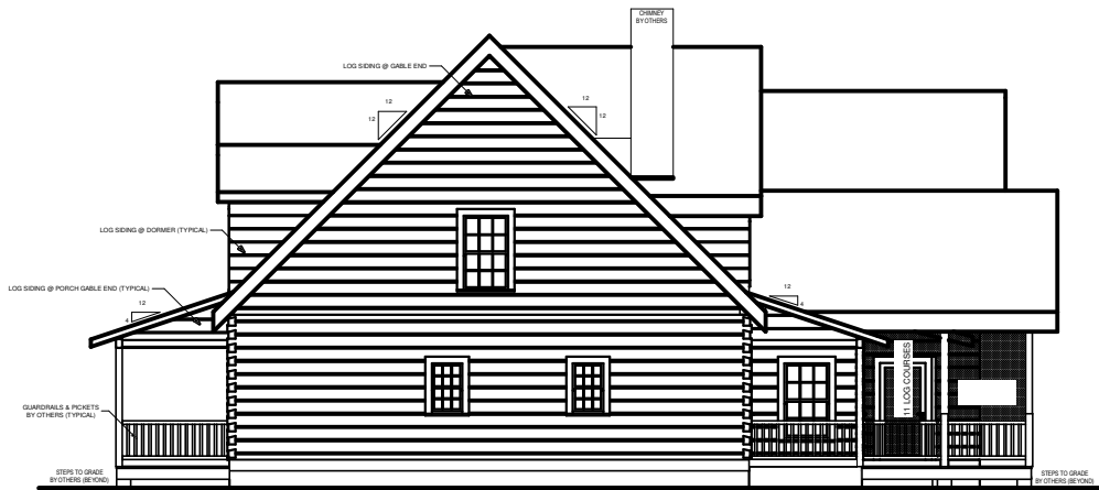
RIGHT ELEVATION
