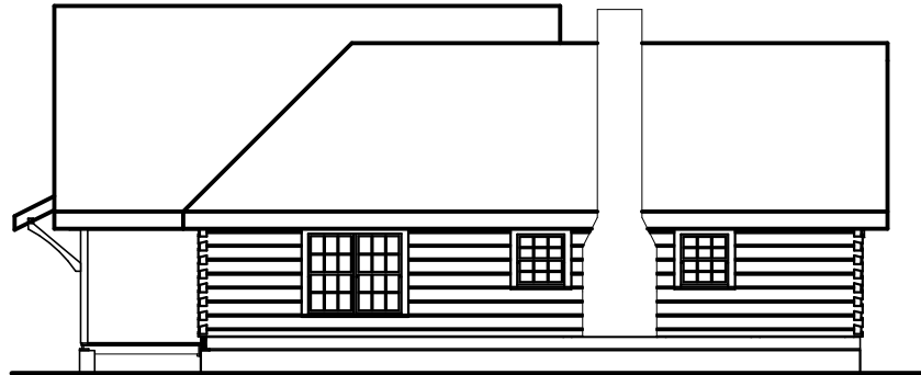
RIGHT ELEVATION
