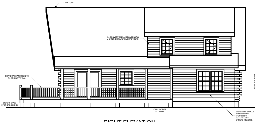
RIGHT ELEVATION
