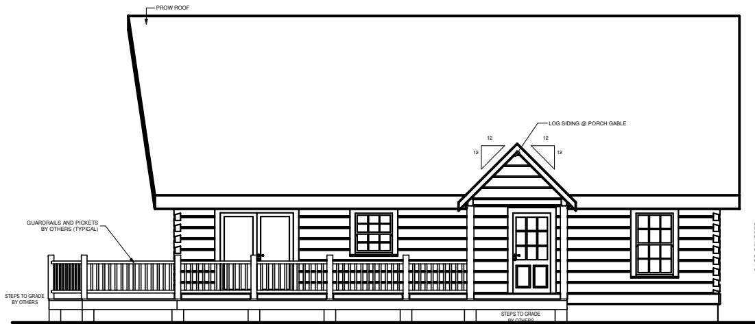
RIGHT ELEVATION
