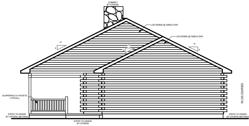
RIGHT ELEVATION
