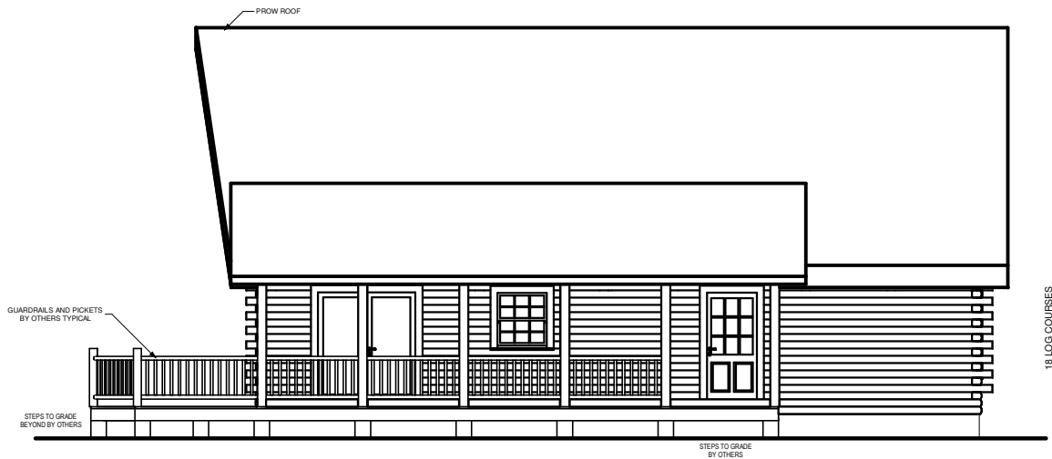
RIGHT ELEVATION
