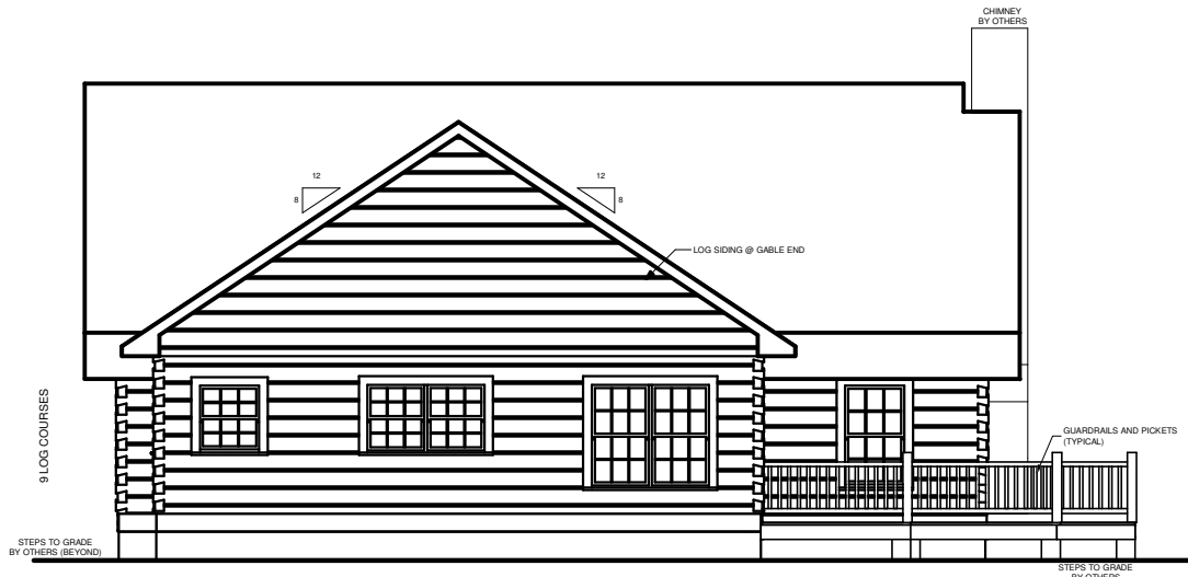
RIGHT ELEVATION
