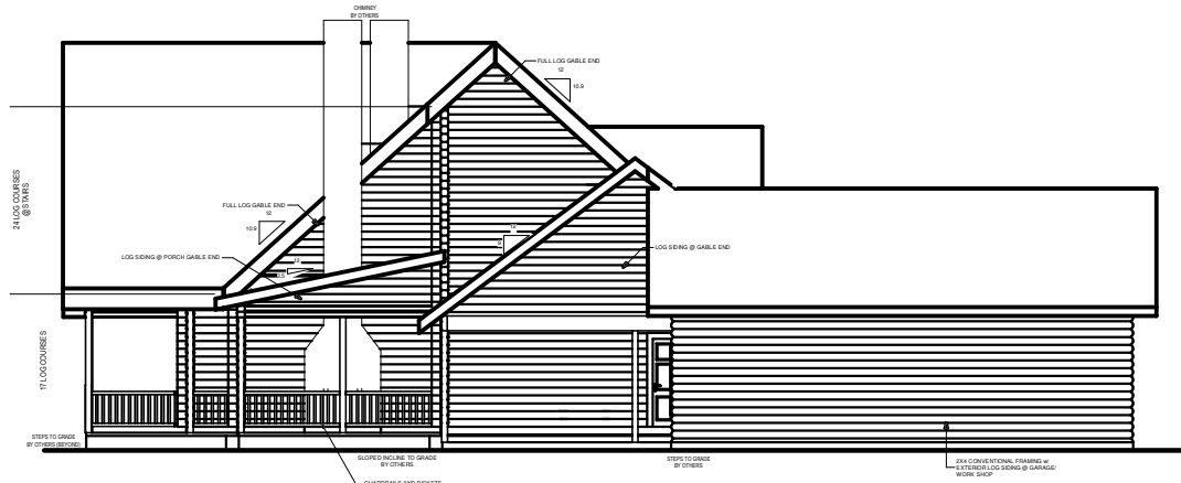
RIGHT ELEVATION
