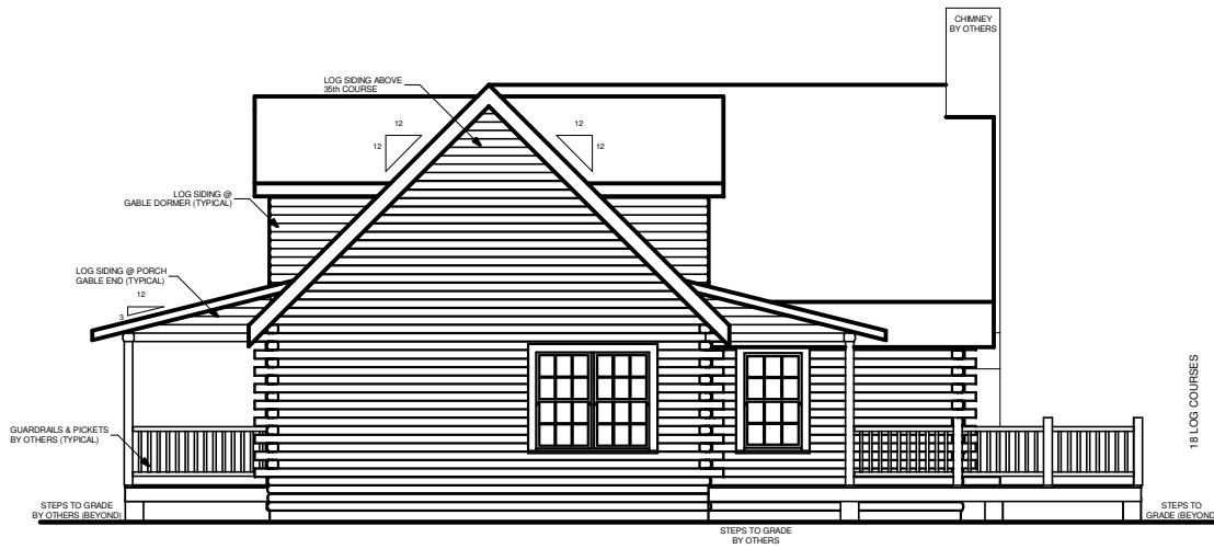
RIGHT ELEVATION
