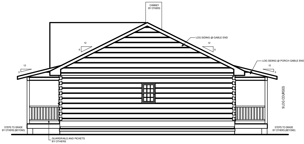
RIGHT ELEVATION
